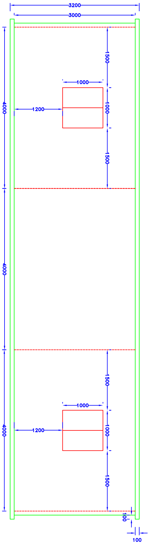
ALZADO POSTERIOR
