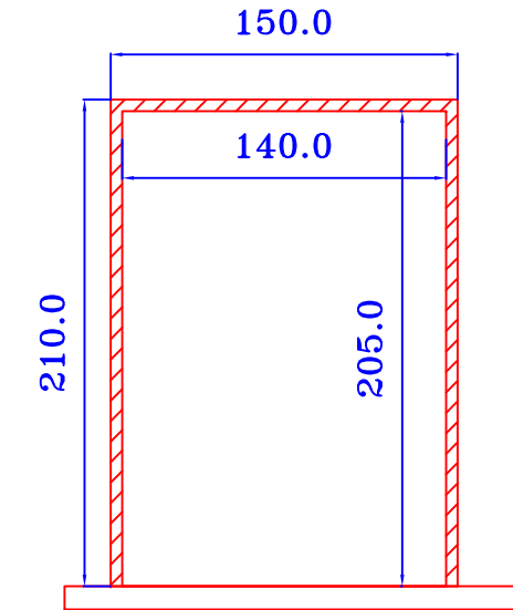
SECCIÓN A-A'
