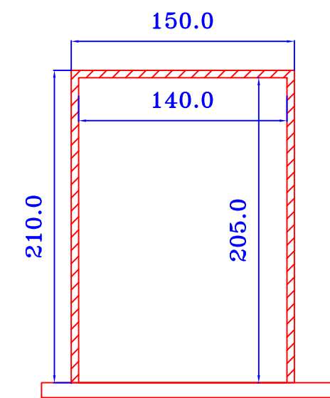
SECCIÓN B-B'
